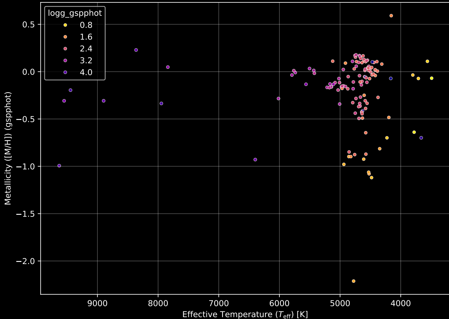
APOGEE DR17 Field: [278-09] Stellar Population Parameters (n= 128)
